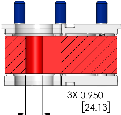
SECTION B-B SCALE 1 : 3
