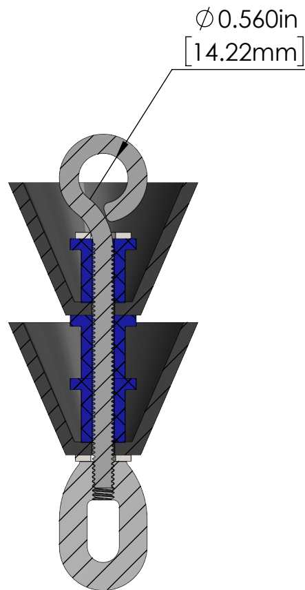
SECTION A-A SCALE 1 : 1.5
