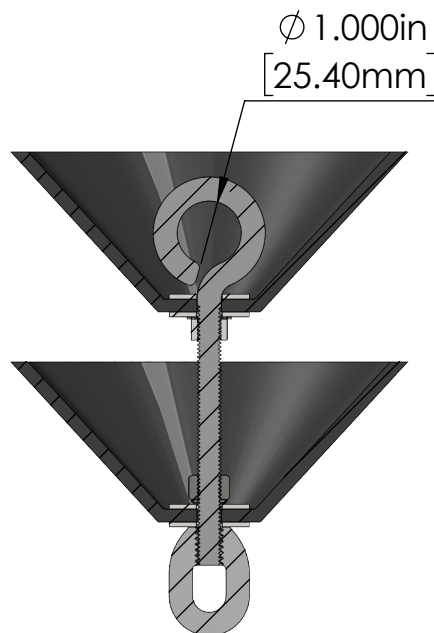
SECTION B-B SCALE 1 : 3
